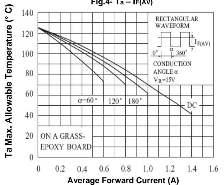
Fig.4- T_a - I_{F(AV)}
